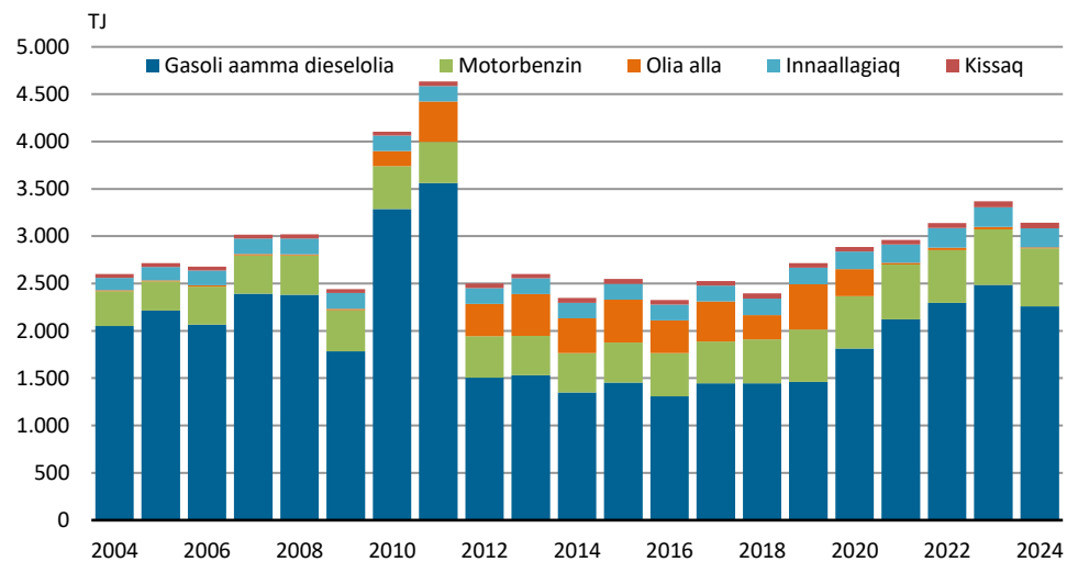
Titartagaq 24. Tunisassiorlutik inuussutissarsiortut nukissiuutinik atuinerat, nukissiuutinut immikkoortiterlugit
