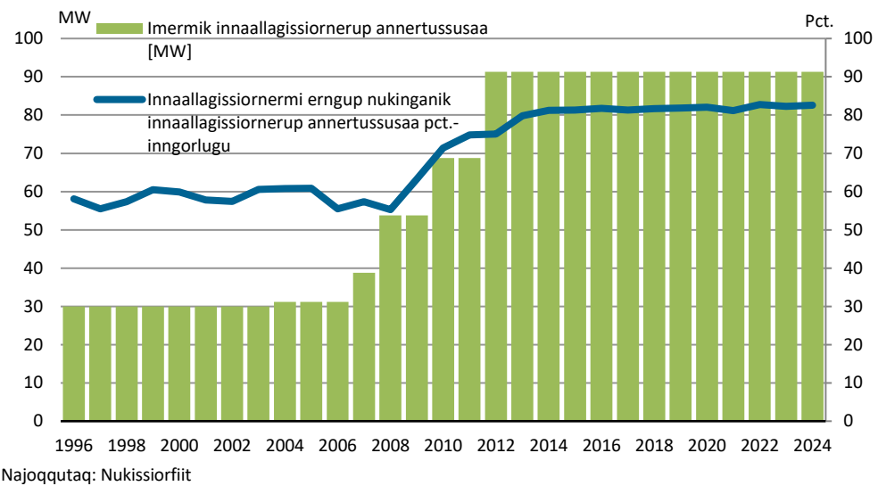
Titartagaq 17. Imermit nukissiuuteqarnerup annertussusia aamma imermit nukissiuutinit innaallagissiornerup annertussusia
