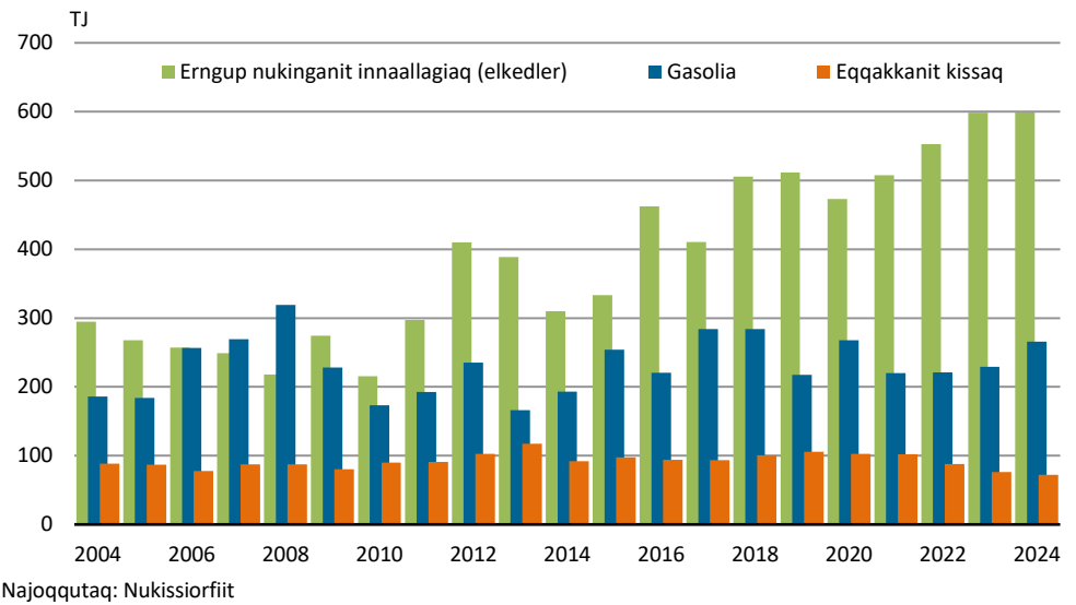
Titartagaq 11. Ungasianit kiassarnermik tunisassiornermi ikummatissanik atuineq
