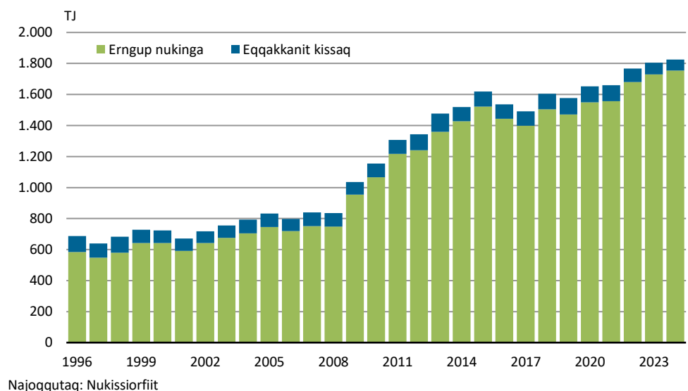
Titartagaq 14. Nukissiuutini pingaarnernik tunisassiorneq
