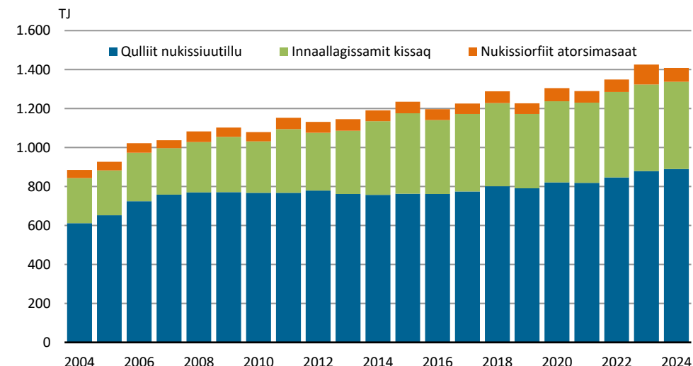
Titartagaq 8. Nukissiorfiit innaallagiamik tunisaat namminneq atorsimasaat ilanngullugu
