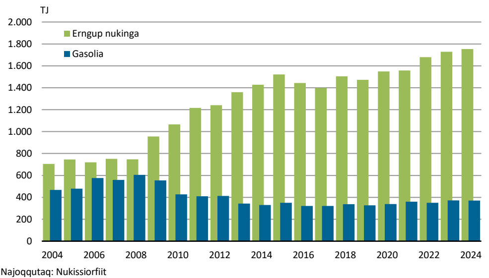
Titartagaq 6. Innaallagiamik tunisassiorneq, ikummatissanut ator neqartunut immikkoortillugit
